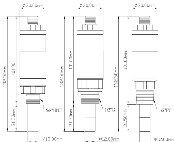
※ 标配—M12-5PIN 2米防水连接线
