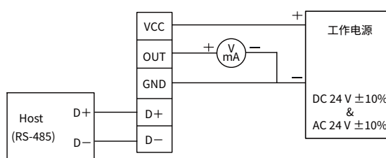
M16 塑料电缆固定座 - 5P端子台 - RS-485
