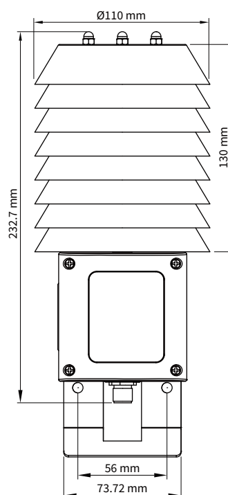
N型: RS-485或模拟讯号
