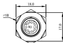
M型(M12-8PIN 接头) RS-485+模拟讯号
